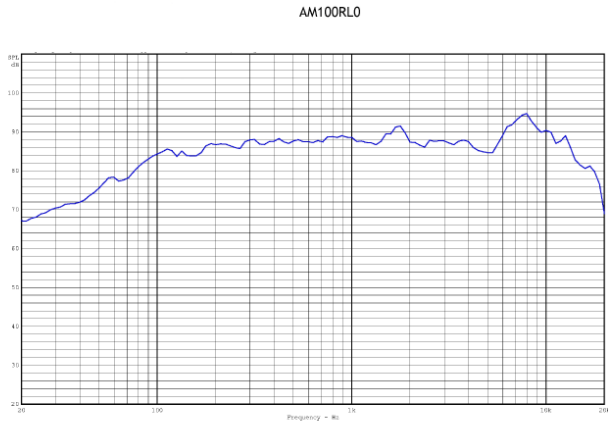
Courbe de réponse @ 2.83V / 1m
